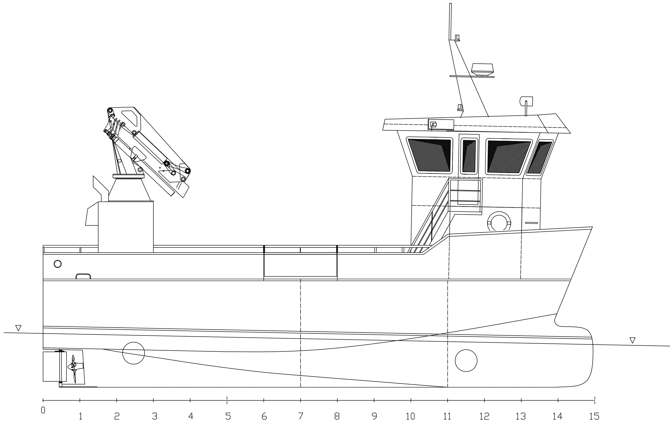
PROFIL
